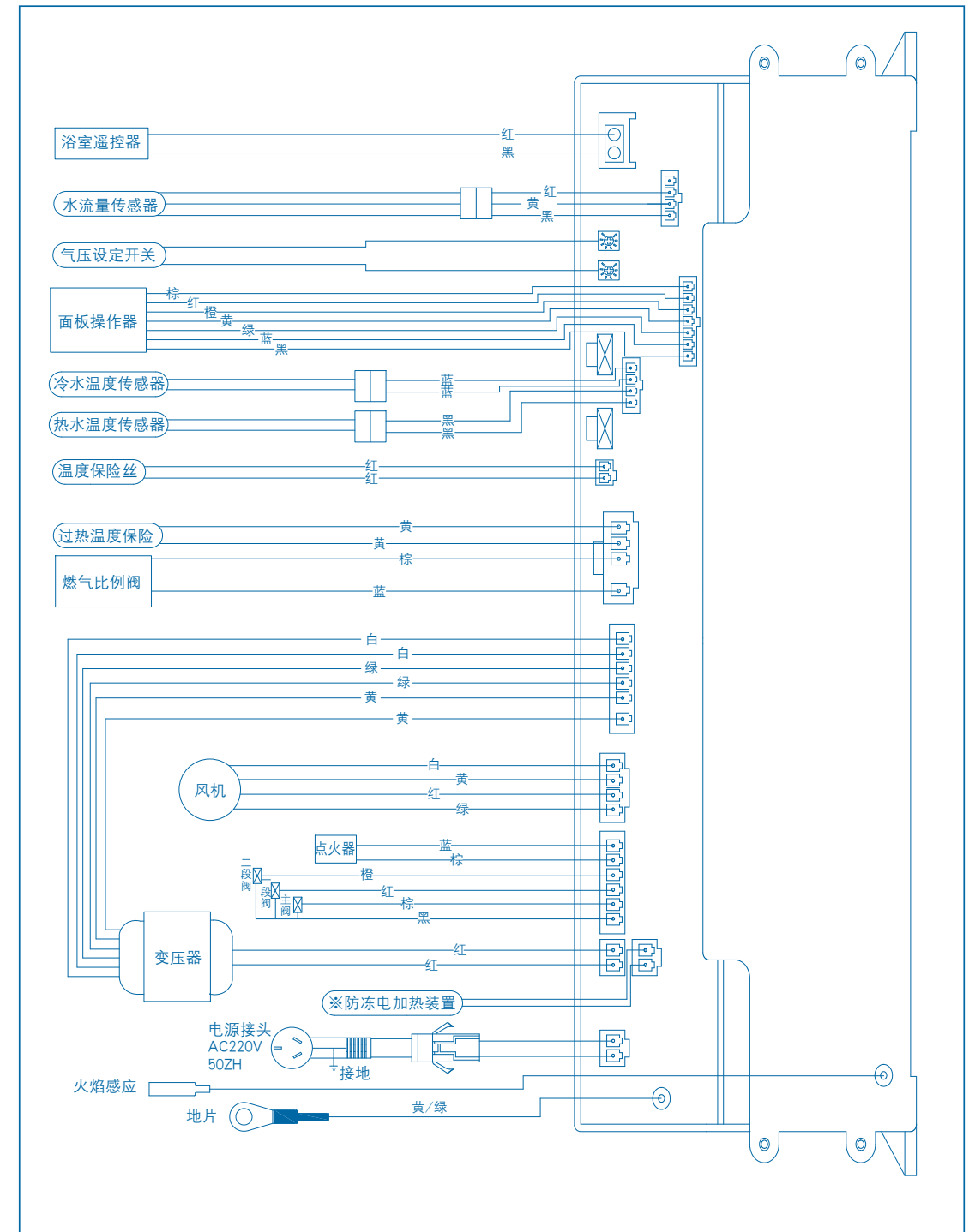
b. Ei7+及Ei6+系列:
