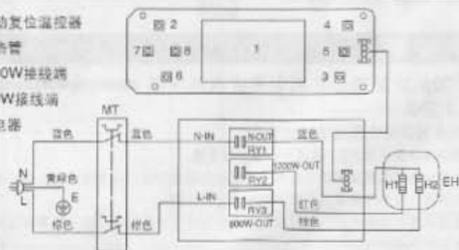
电气原理图
