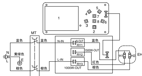
R3 机型 电气原理图
