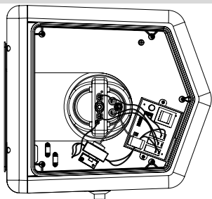
R3机型接线图
