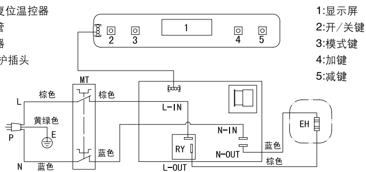
电气原理图
