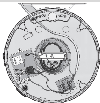
接线图
