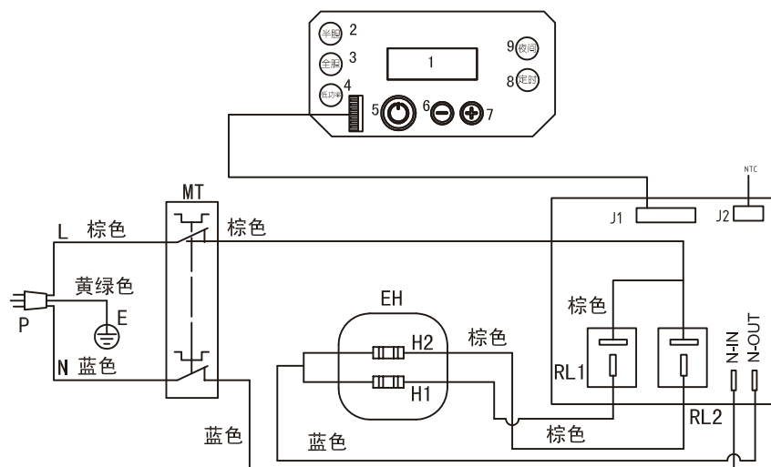
电气原理图
