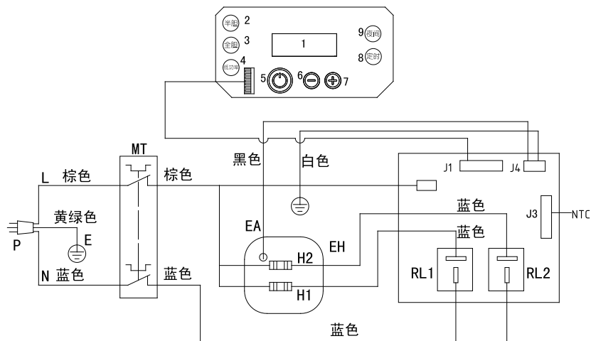
电气原理图
