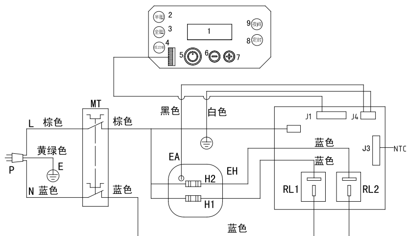
电气原理图
