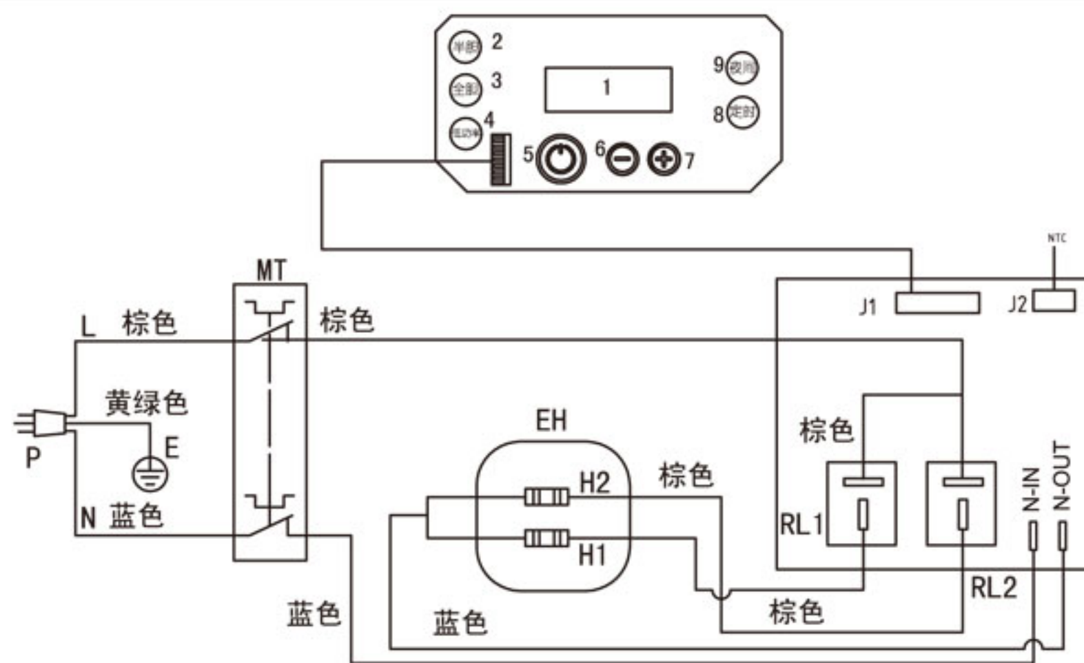
电气原理图
