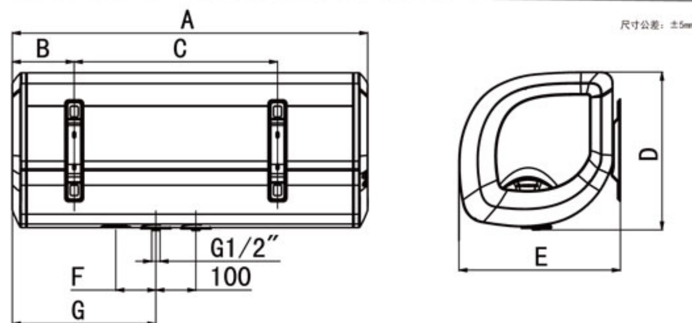
EHT50E2.5AG EHT60E2.5AG EHT60SE2.5AG EHT80E2.5AG
