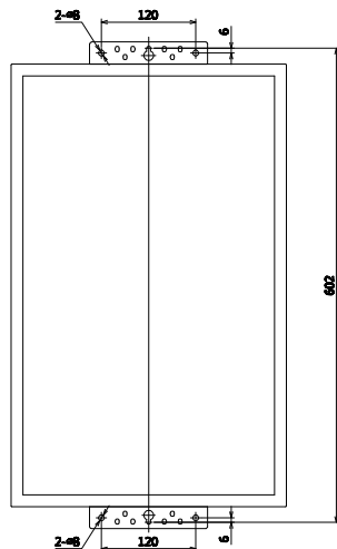
安装孔位示意图
